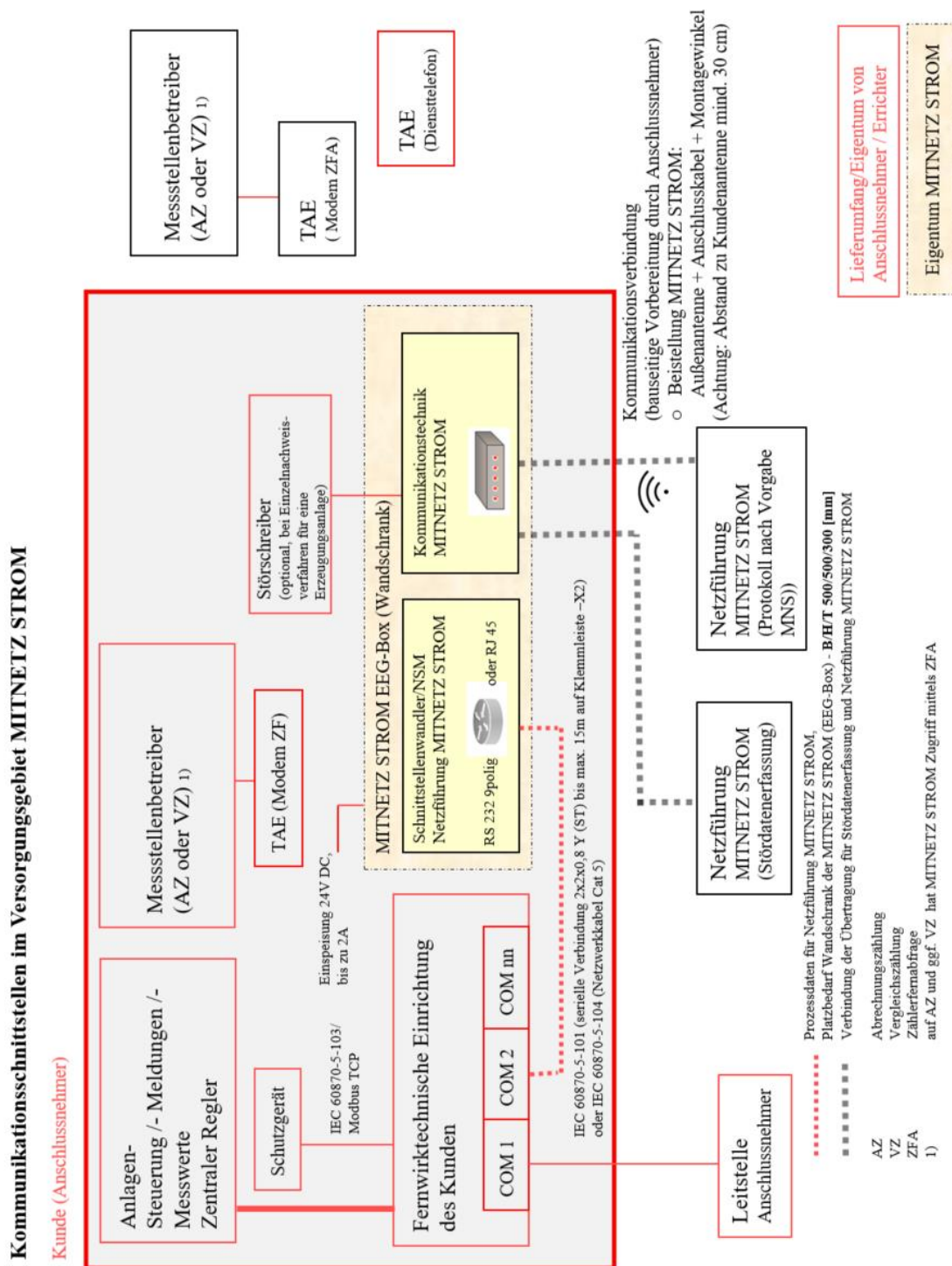
Abb. 20: Kommunikationsschnittstellen
