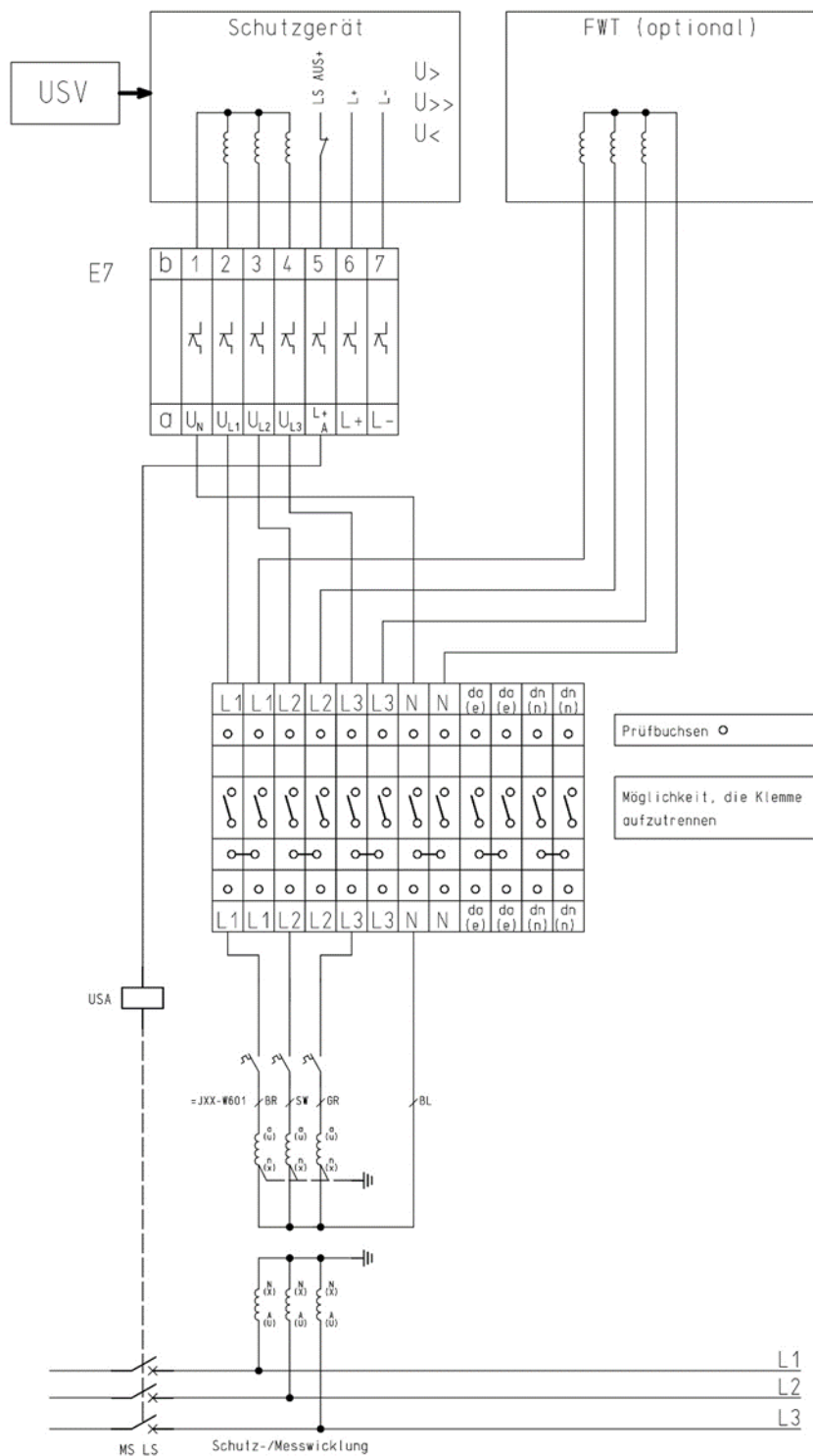
Abb. 48: Wandlerverdrahtung Anbindung übergeordneter Entkopplungsschutz / Fernwirkgerät
