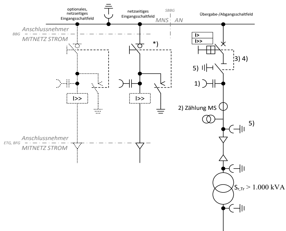
Abb. 24: (ehemals D1b): \leq 20 -kV-Anbindung mit einem Abgangsfeld; Transformator > 1 MVA
